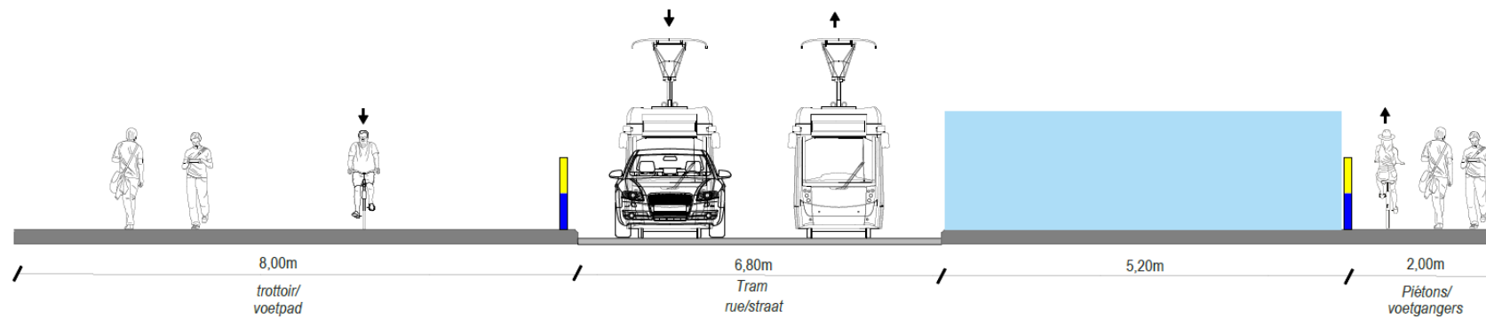
Situation Chantier - Werfsituatie
